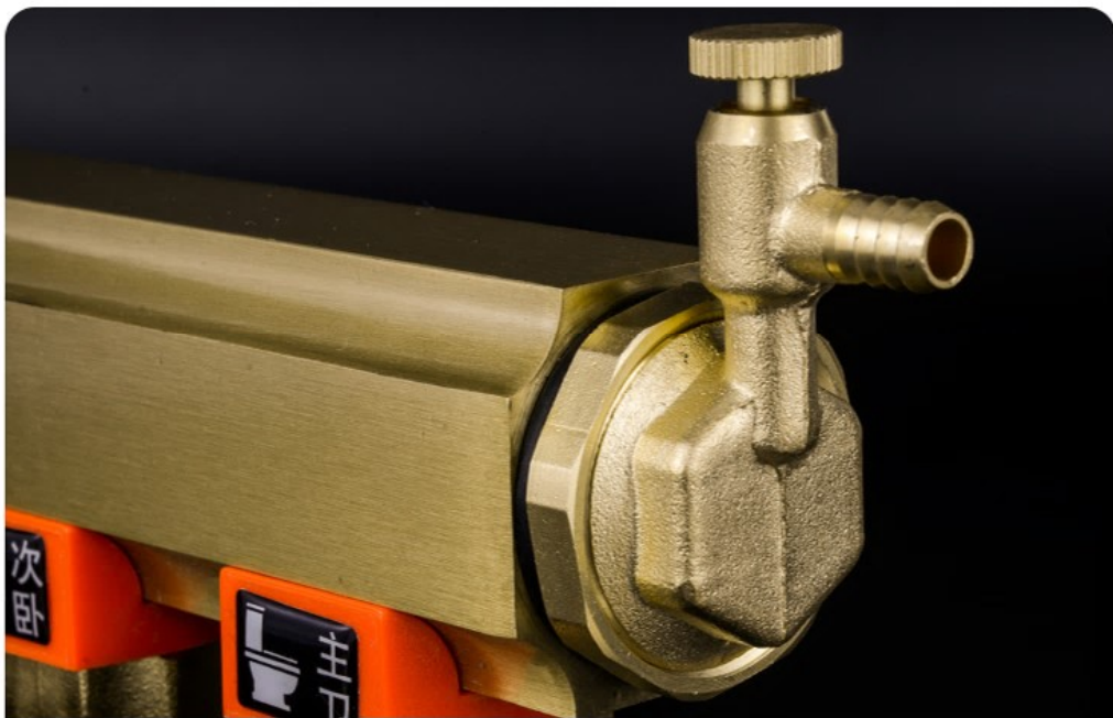
管堵一体排气阀 01 Details
